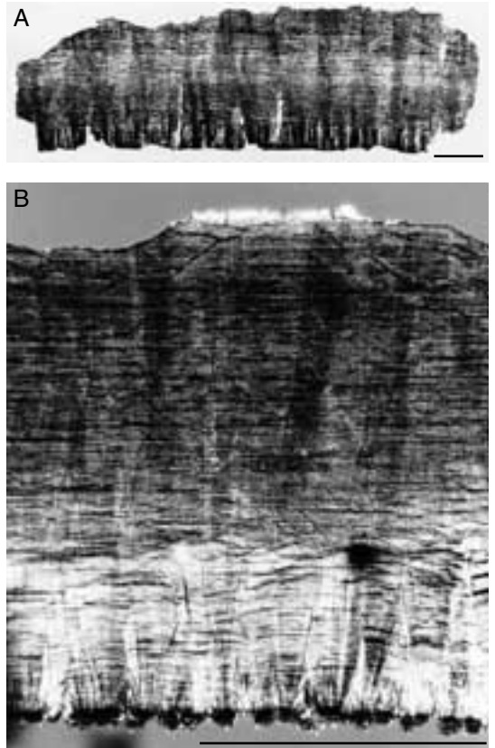
FIG. 3. — Lames minces réalisées à la demande de Paul Gervais dans des fragments de coquille d'œuf d'oiseaux en 1876. Collections du Laboratoire d'Anatomie comparée du Muséum national d'Histoire naturelle, Paris ; A, œuf d'autruche, coupe radiale ; B, œuf d' Aepyornis , coupe radiale. Echelles : 1 mm.
